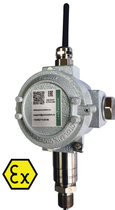
Рис. 1. Датчик давления со встроенным GSM-модемом «Логгер PROMODEM 122.B2M» во взрывозащищенном Exd-корпусе
